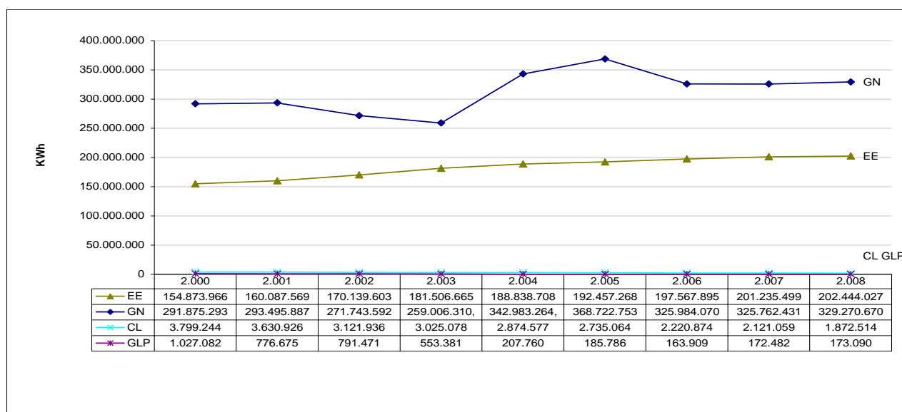
Gràfic 9. Consums finals del sector domèstic de Lleida per fonts.
