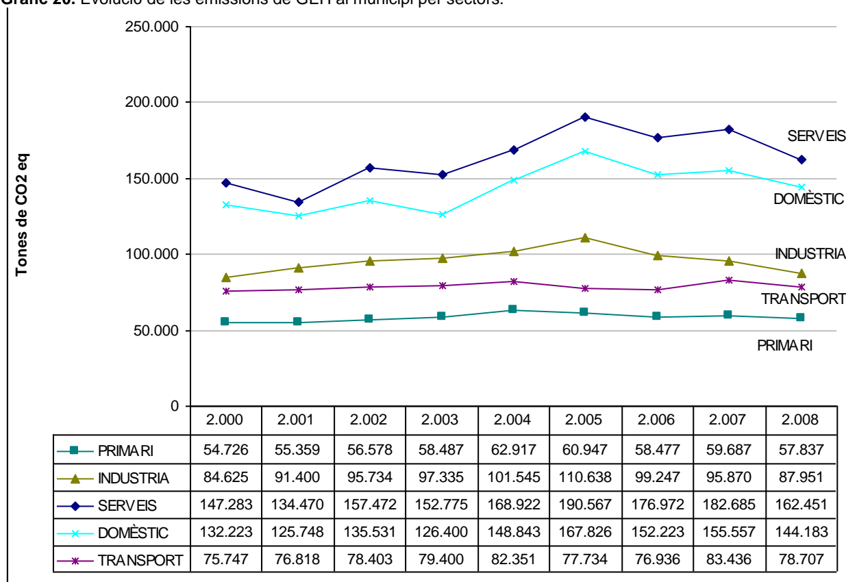
Gràfic 20. Evolució de les emissions de GEH al municipi per sectors.
